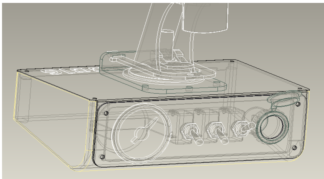
Modèle 2, face avant pour 1 mano, 3 inter à levier et une embase allume cigare (Représenté également avec support bride GPS)
